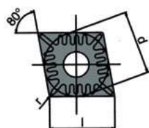
CNMG insert
