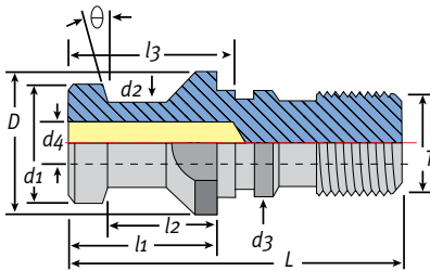
DIN 69871B
