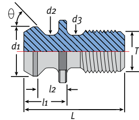
ANSI Style
