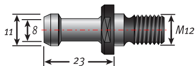
BT30 – 45°
