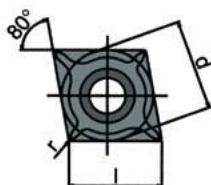
CCMT insert
